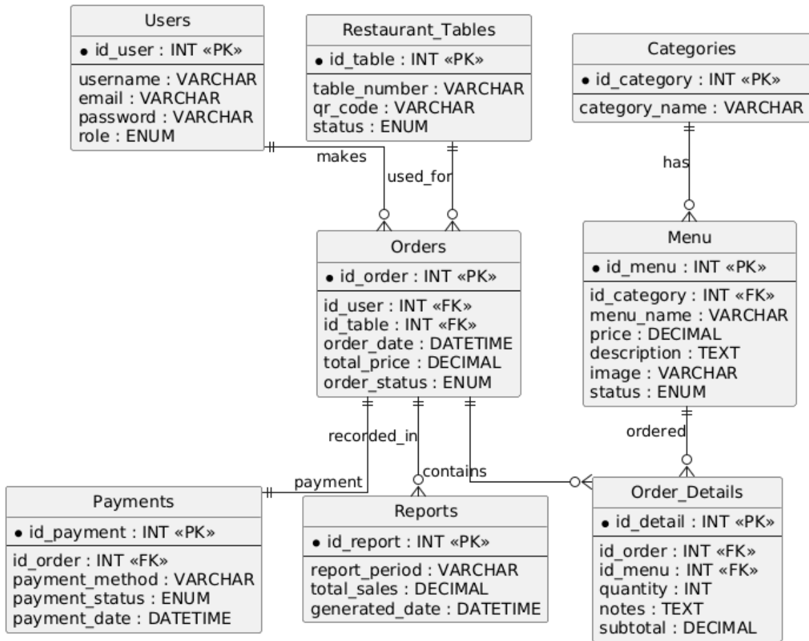
(Gambar ERD)
